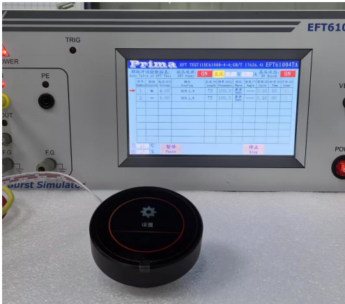
图 6-4 群脉冲测试图
