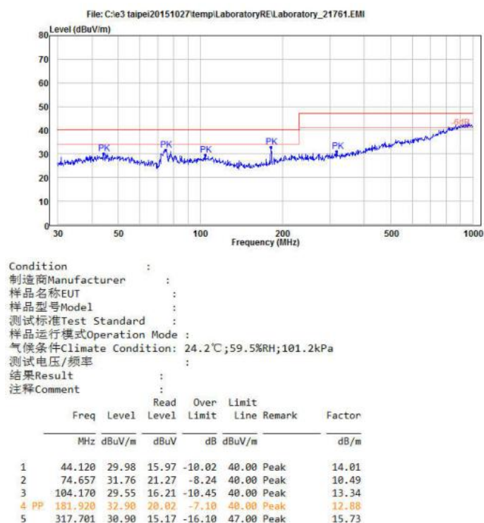
图 6-7 辐射测试垂直方向
