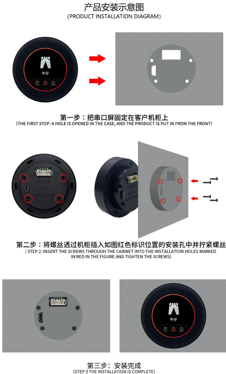
图 2-1 安装示意图
